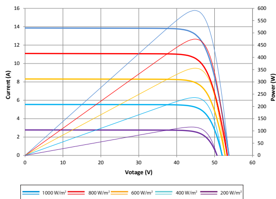
电流-电压 &amp; 功率-电压曲线图 (590S)
